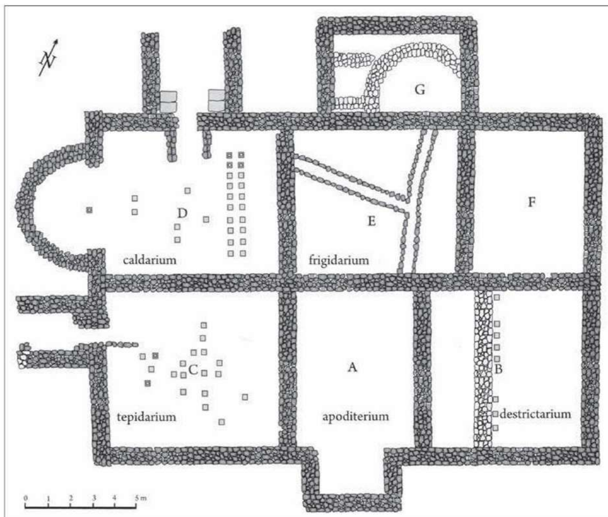
Fig. 4. Planul thermei A de la Ilișua.
